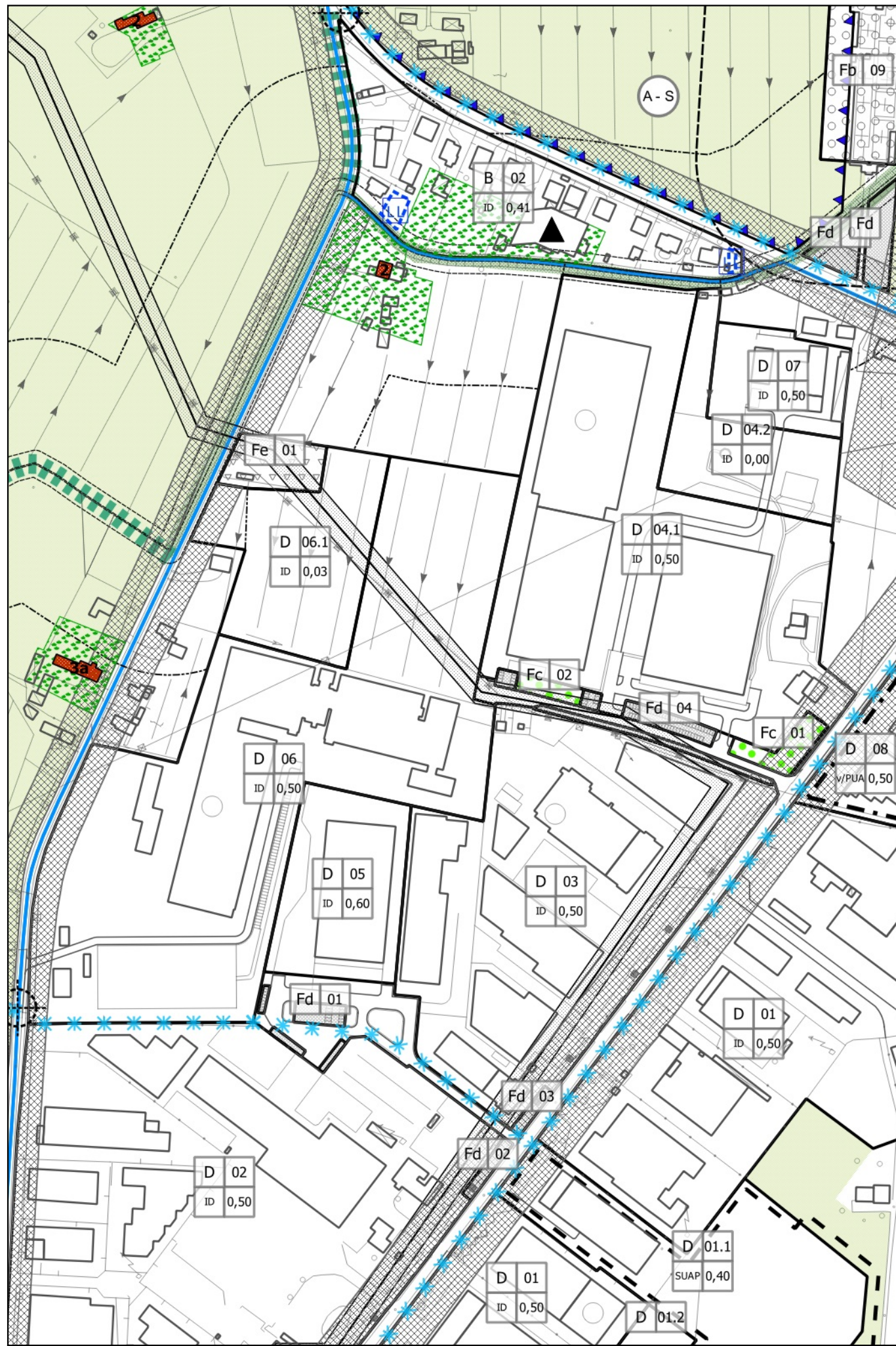
PI VARIANTE - estratto Tav. 3.1 scala 1:2.000
